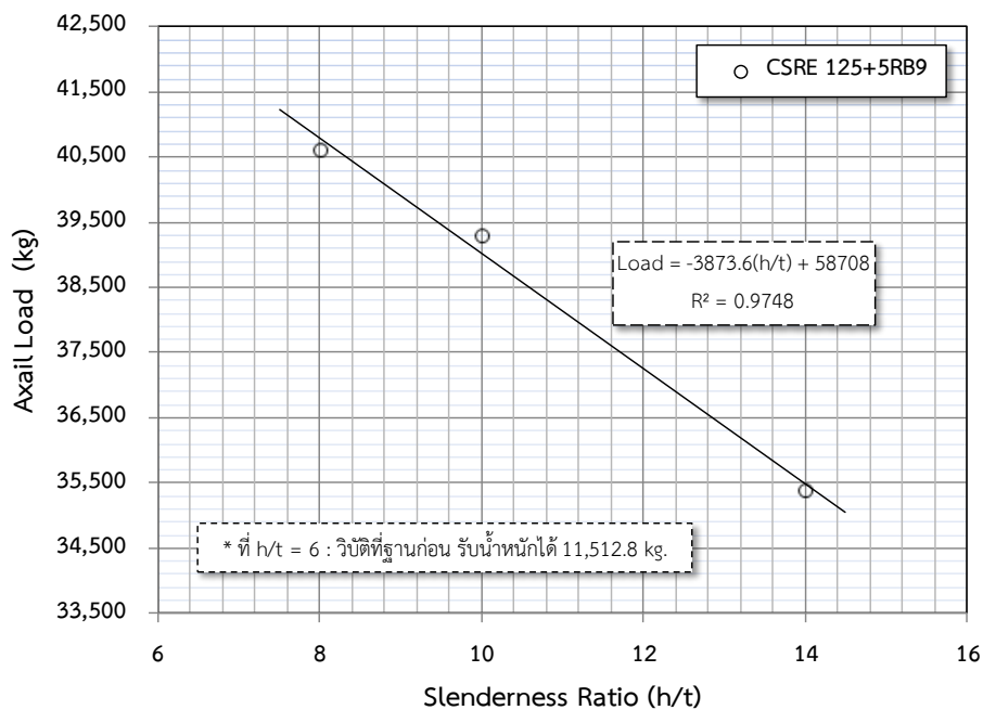
รูปที่ 4 : ความสัมพันธ์ระหว่างค่าอัตราส่วนความชะลูดของผนังกับแรงกดอัด
