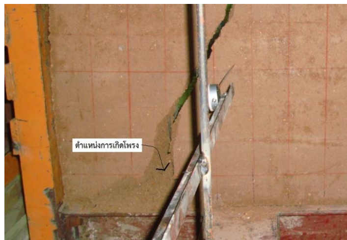
รูปที่ 5 : ด้านล่างของผนังดินซีเมนต์บดอัดเกิดเป็นโพรง
