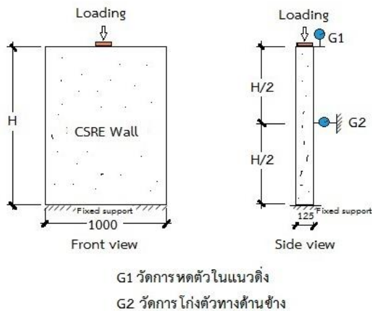
รูปที่ 3 : รูปแบบการทดสอบแรงกดอัดของผนัง
